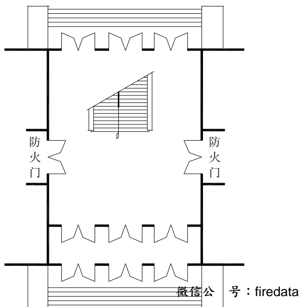
图 5 扩大封闭楼梯间示意图
